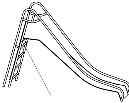
2x Verschraubung Sicherheitschraube-ISO 7380-M8x20-A2
