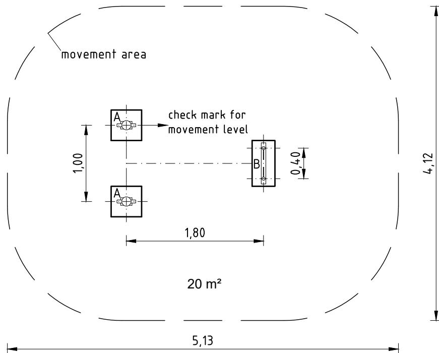
type A 1:20
