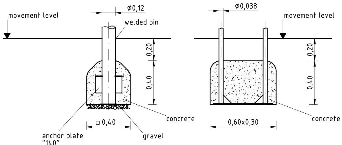
type A 1:20
