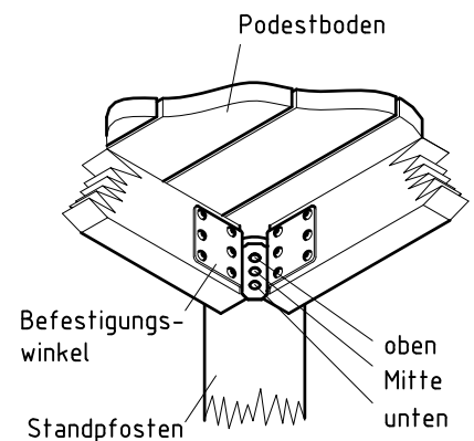
Podestbodenbefestigung 1:10
